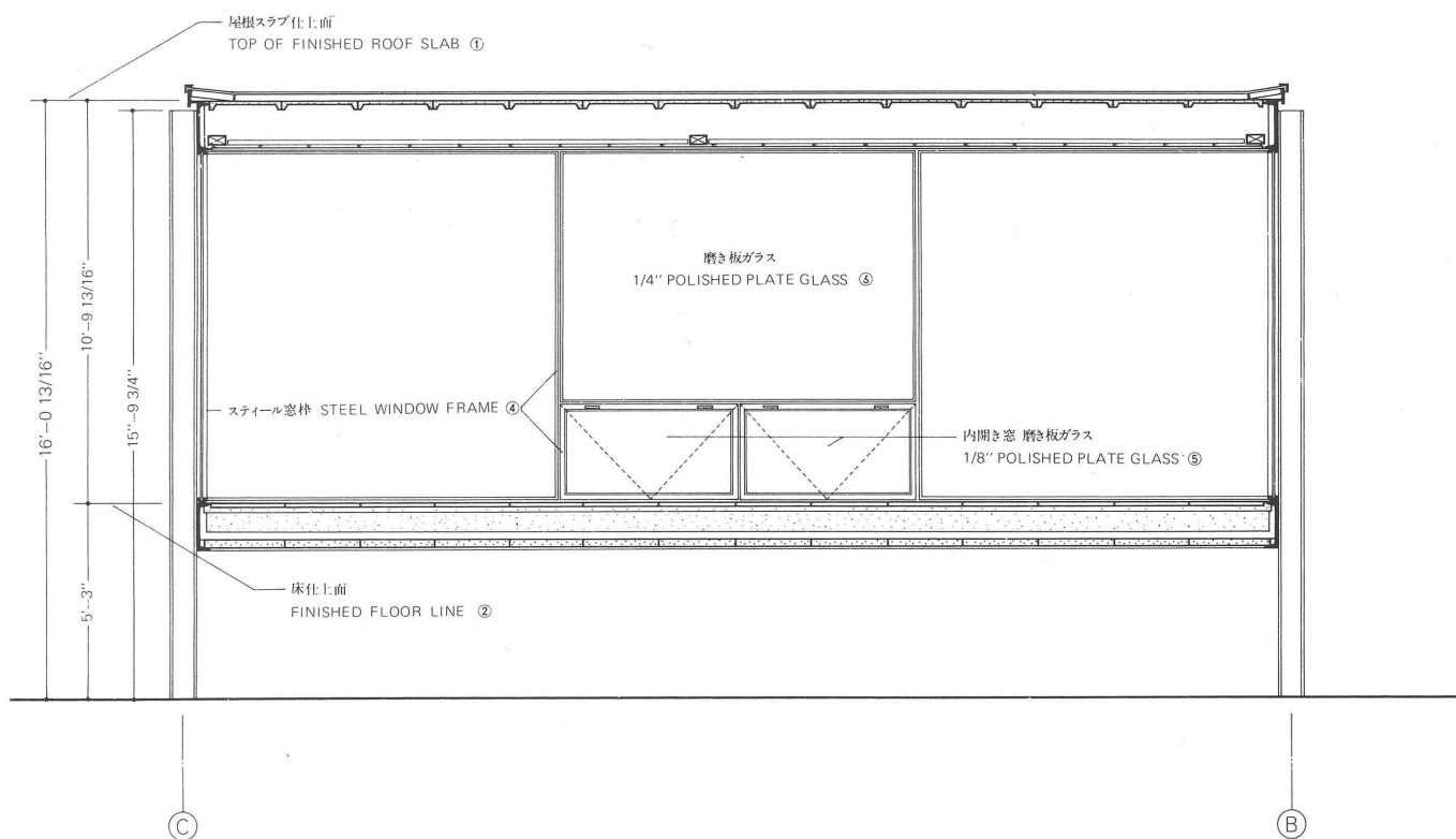
横断面図 柱③と④の間を切って東を見る Cross Section between Column Lines ③ & ④ Looking East
