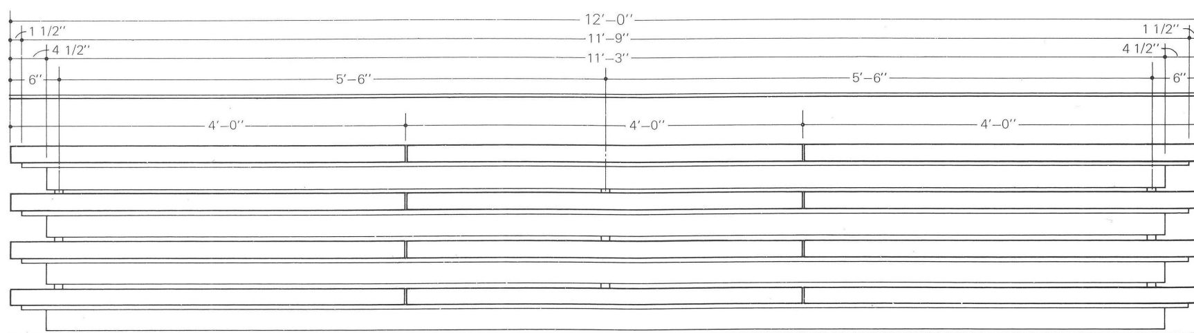
階段 B 立面図 Elevation of Stair B
