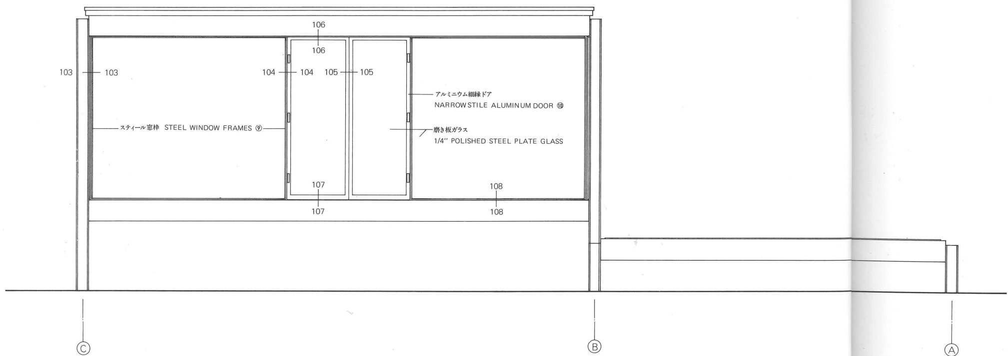
西立面図 West Elevation
