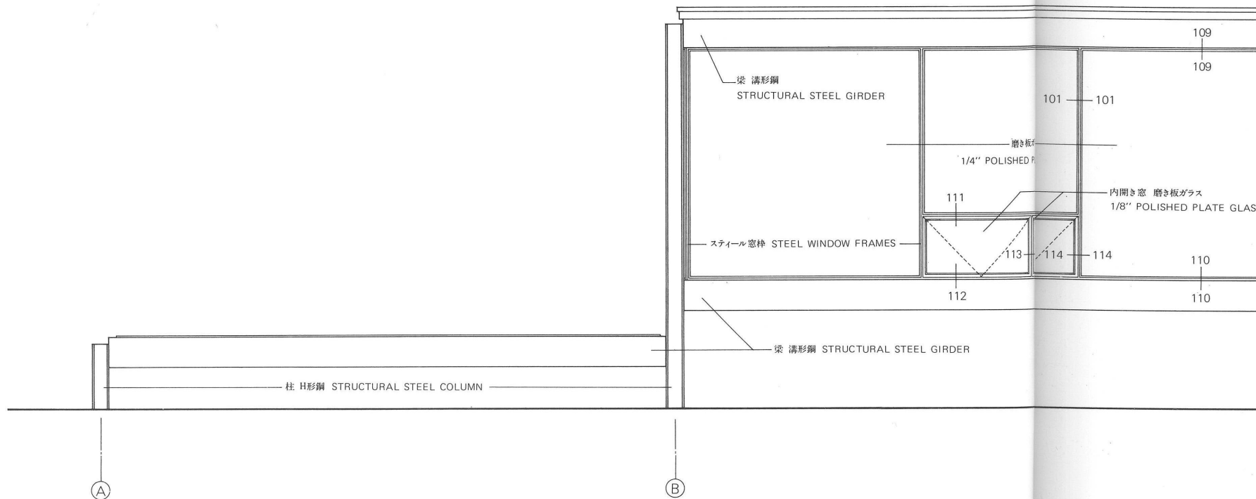
東立面図 East Elevation
