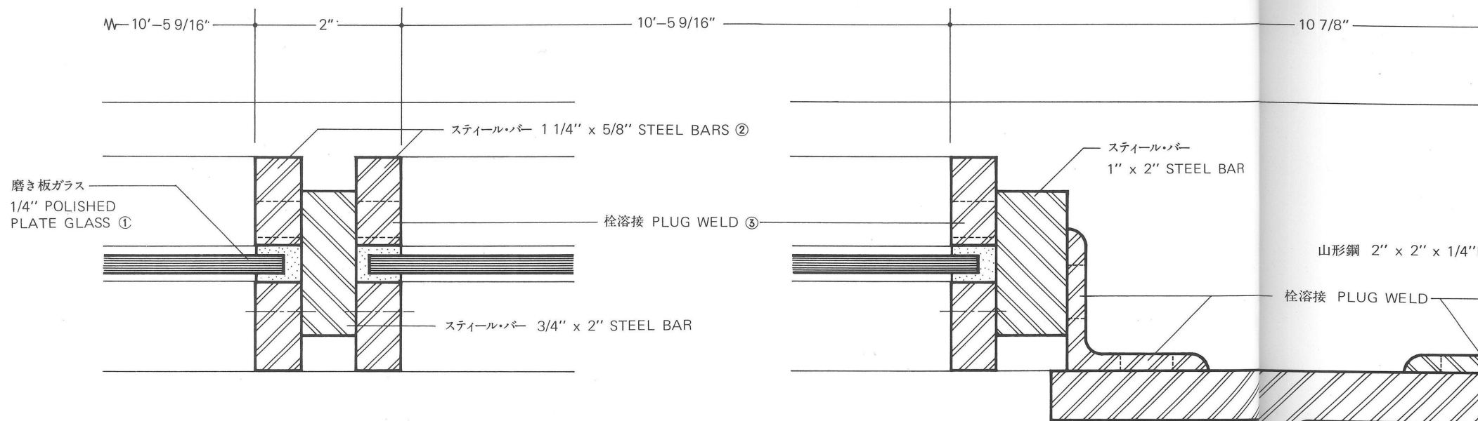
断面図 Section 101
